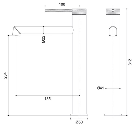
Mértékegység: mm
